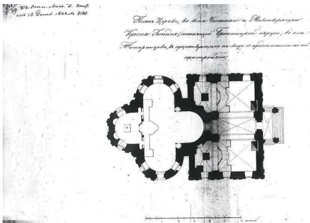
Проект пристройки трапезной, 1844г. ЦИАМ, ф.203, оп.748, д.255
