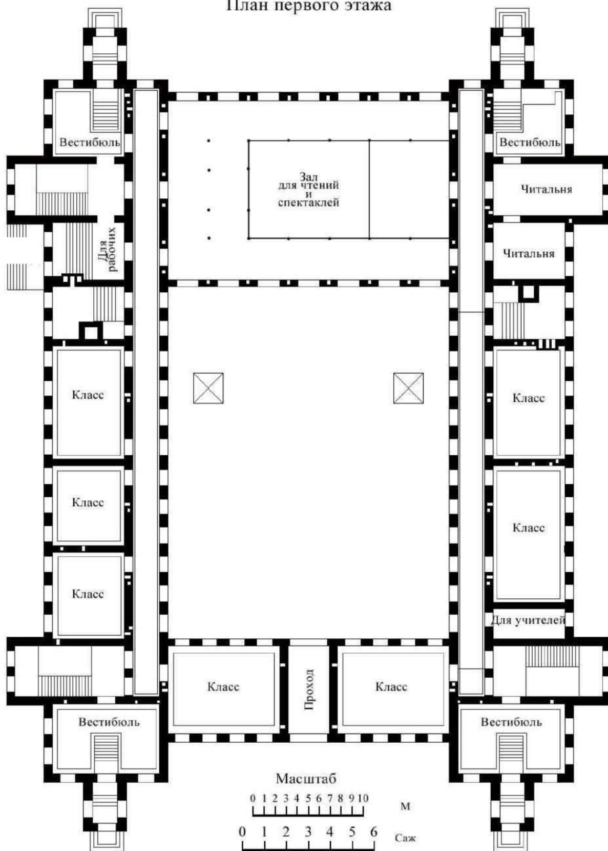
План первого этажа
